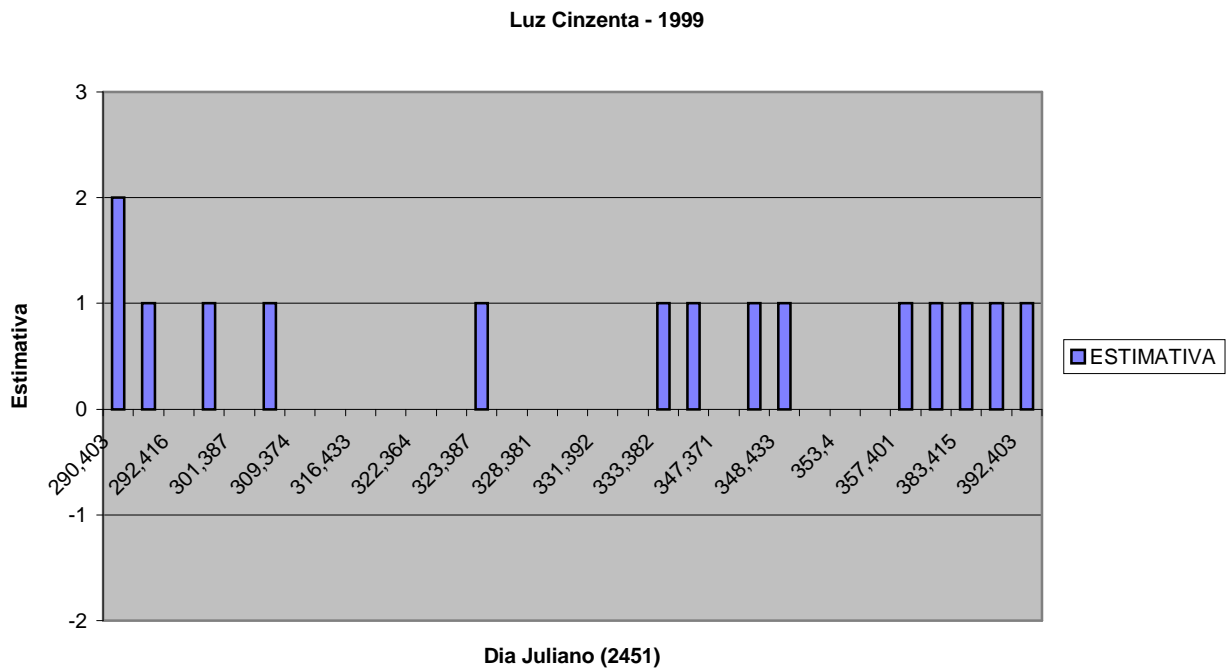
Figura 2: Gráfico da Estimativa x Dia Juliano para a elongação citeriana de 1999
